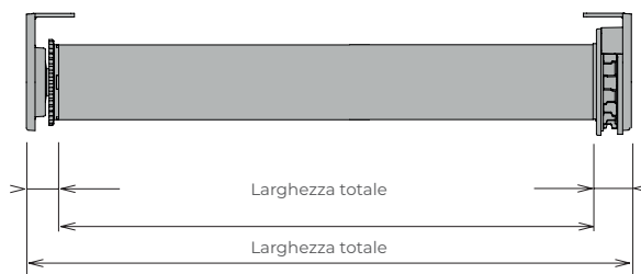
Contrappeso visto in alluminio
