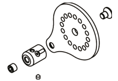
Accessori per guida cavo orientabile
